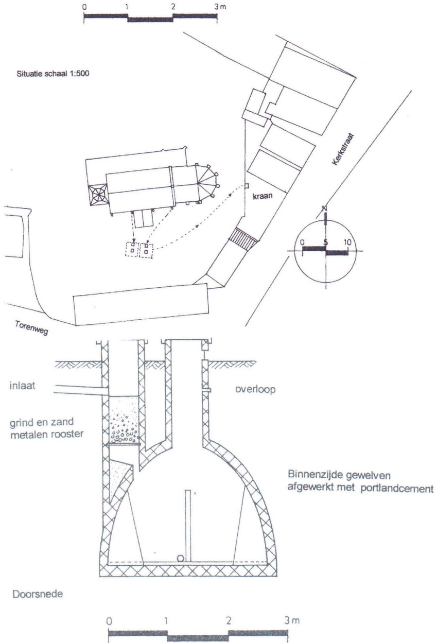
De waterput bij de Willibrordkerk, (tekening Ir. H.N. Karsemeijer)
